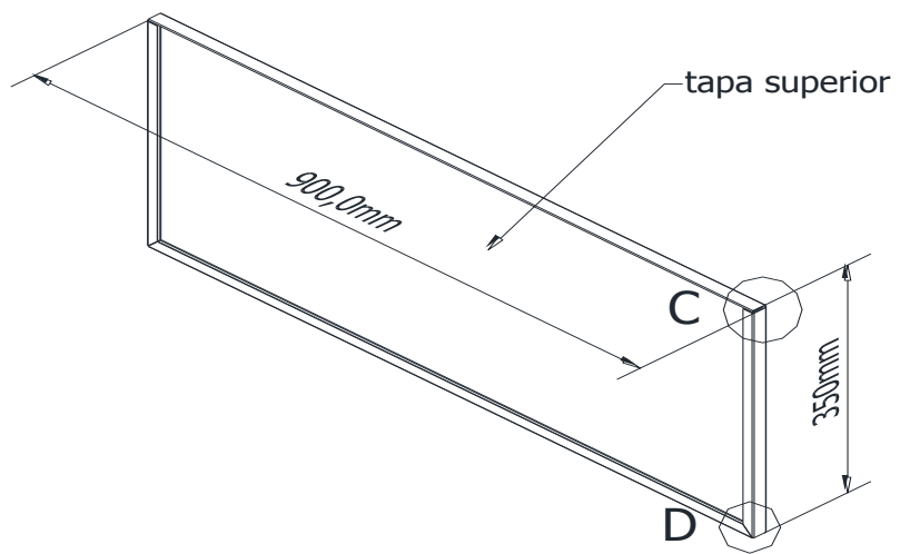
Tapa superior y desarrollo de tapa superior.-
