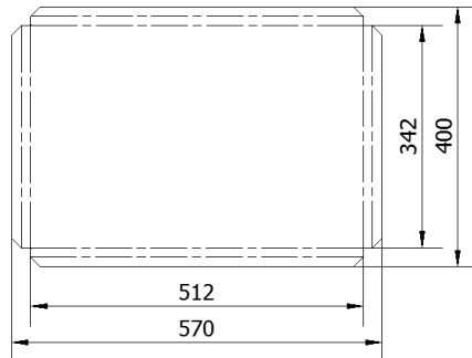
Desarrollo
