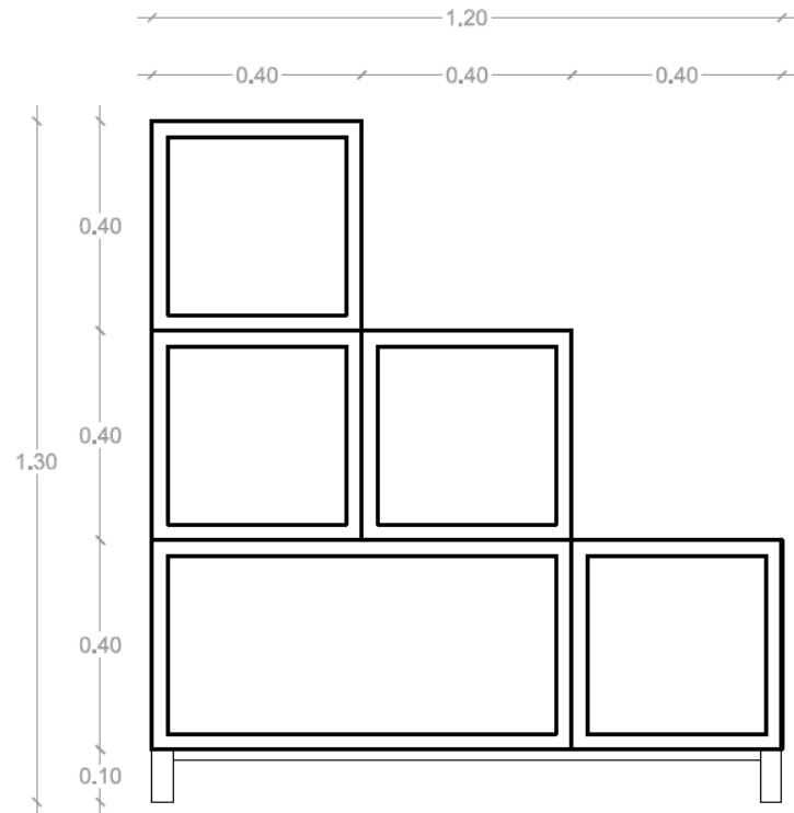
Vista frontal Escala — 1:15
