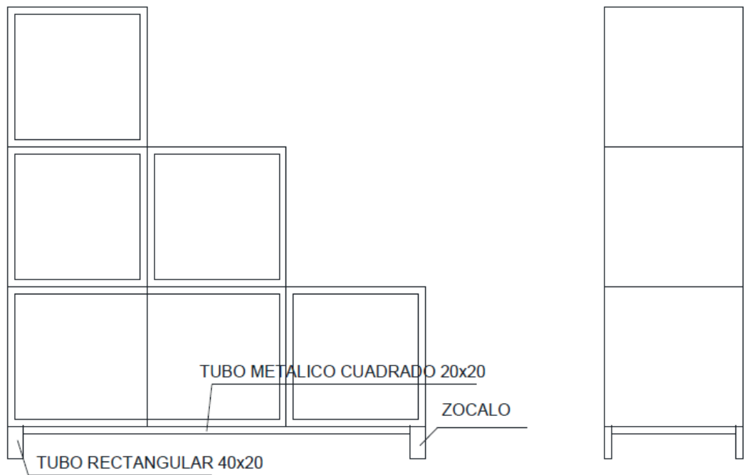
Vista frontal Escala — 1:15
