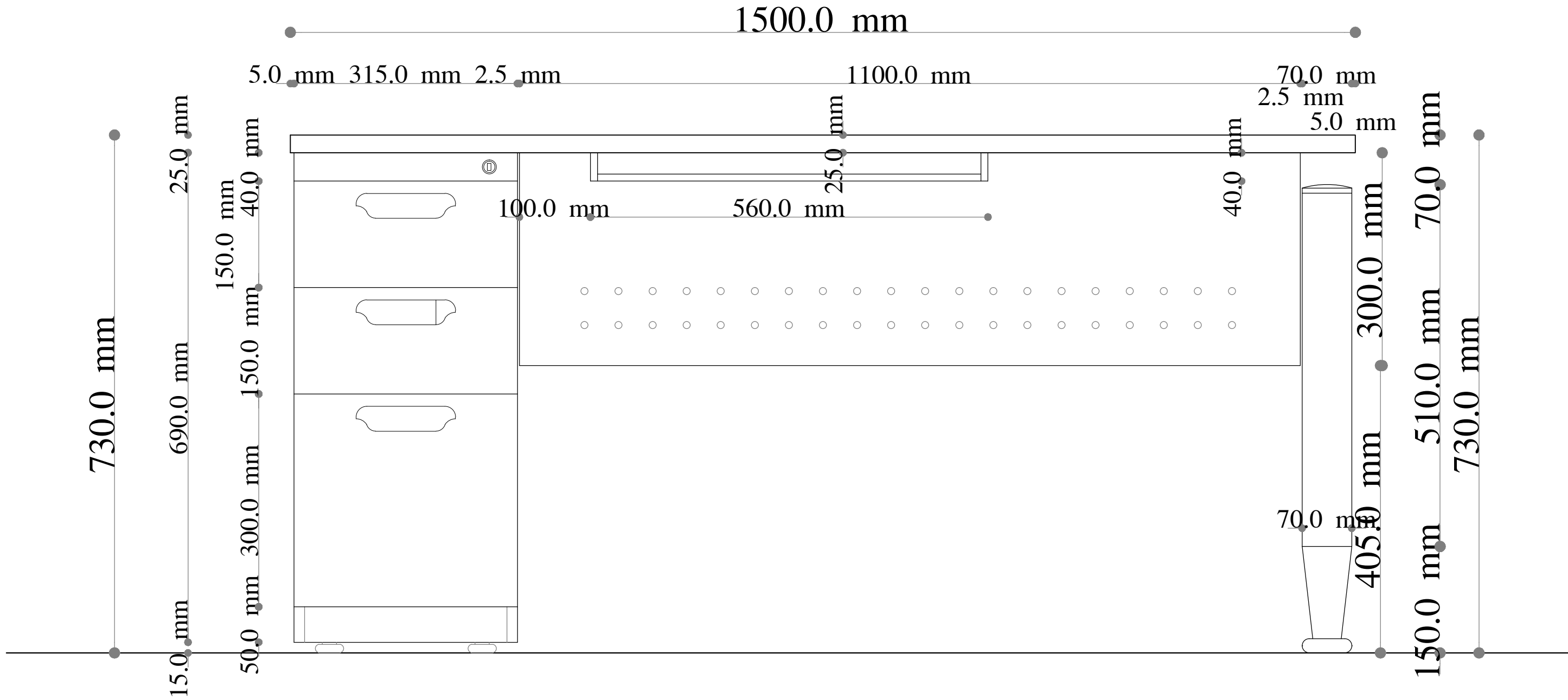
Alzado Frontal
